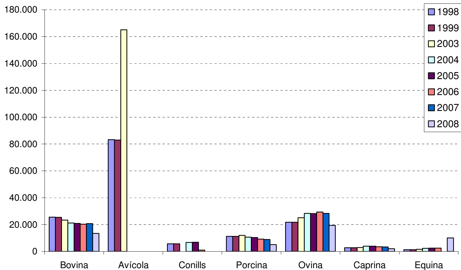
Gràfic 1. Evolució de la cabana ramadera a Menorca dels anys 1998 i1999 i del 2003 al 2008. Graphic 1. Livestock in Minorca 1998, 1999, 2003-2008.
