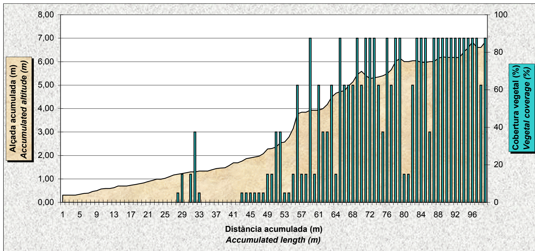
Gràfic 2. Perfil dunar i cobertura de la vegetació del Transsecte 4 de Tirant Graphic 2. Dune profile and vegetal coverage of the Tirant Transect 4
