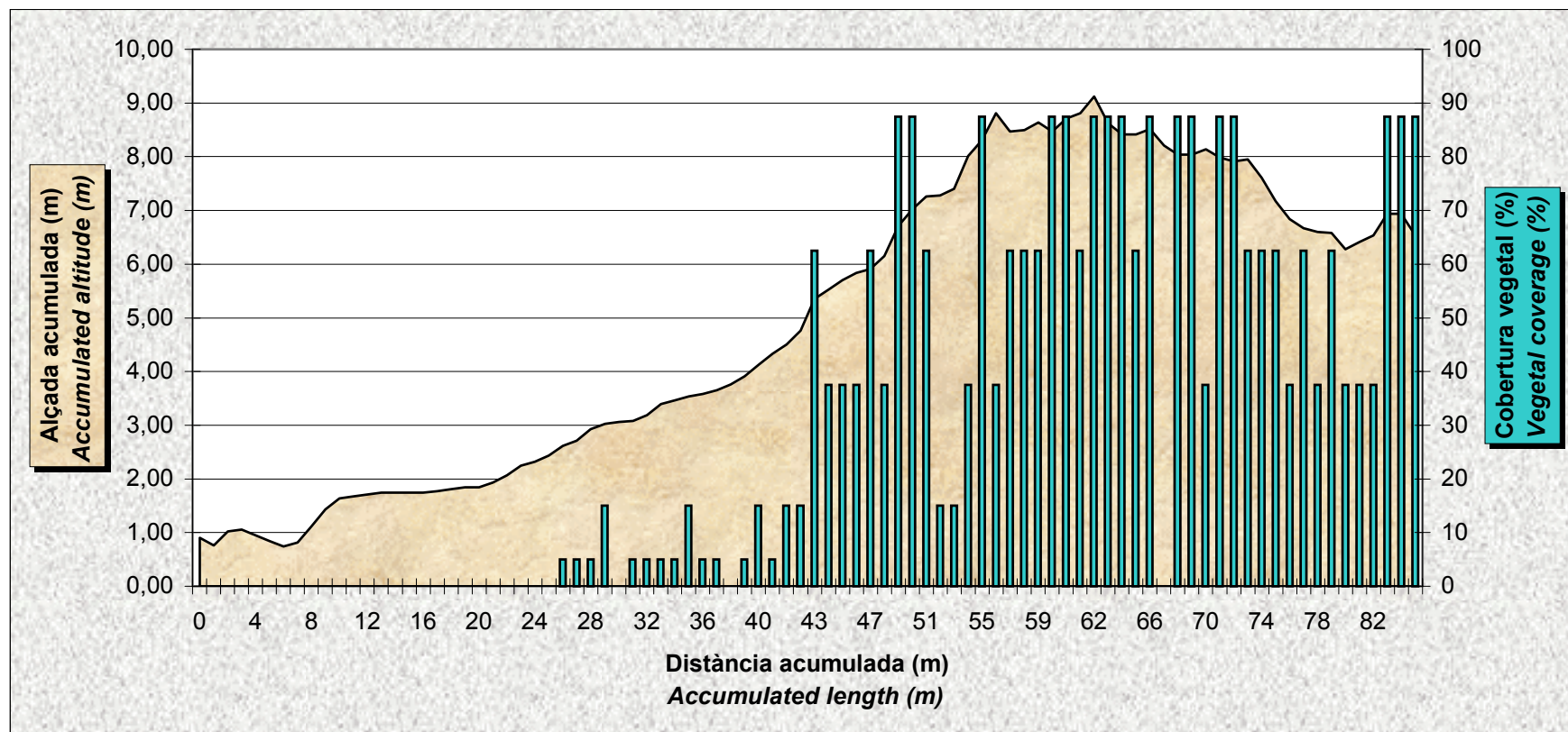
Gràfic 1. Perfil dunar i cobertura de la vegetació del Transsecte 2 de Tirant Graphic 1. Dune profile and vegetal coverage of the Tirant Transect 2
